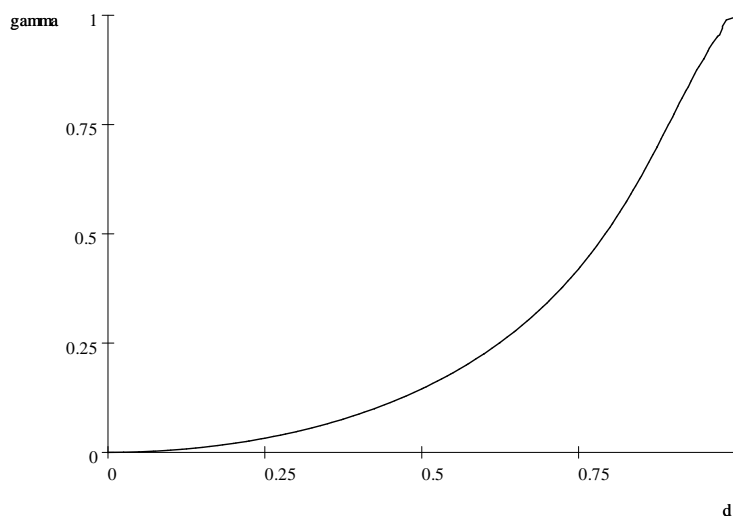
Graf til g(d, \gamma) = (p_{i,tt}^{Nash} - p_{i,lp}^{Nash}) .
