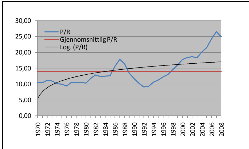
FIGUR 21: P/R-KOEFFISIENTER FRA 1970-2008.
