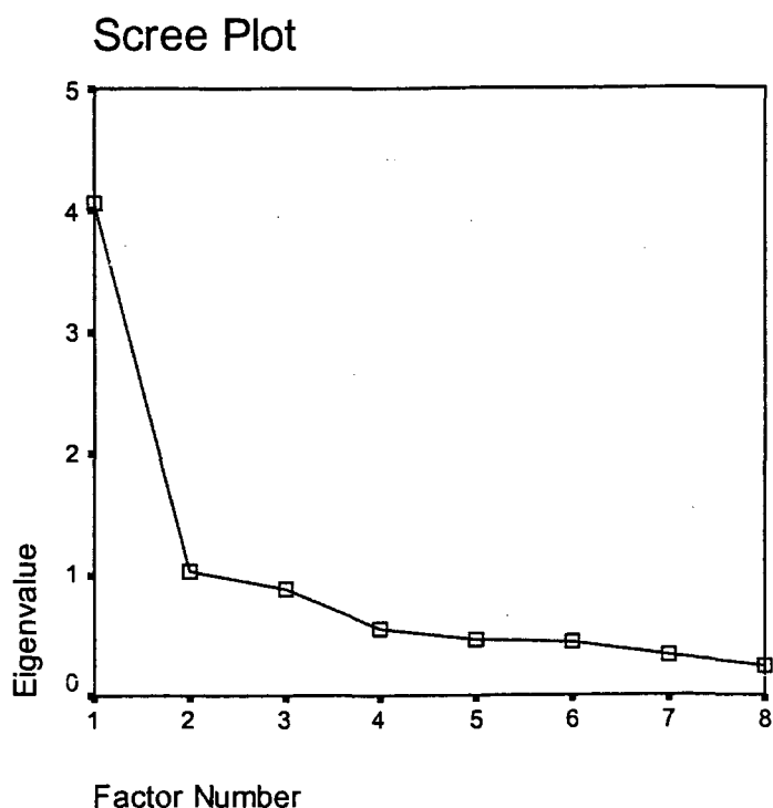
Figur 6.4 Scree plot Overordnede lover, regler og avtaler
