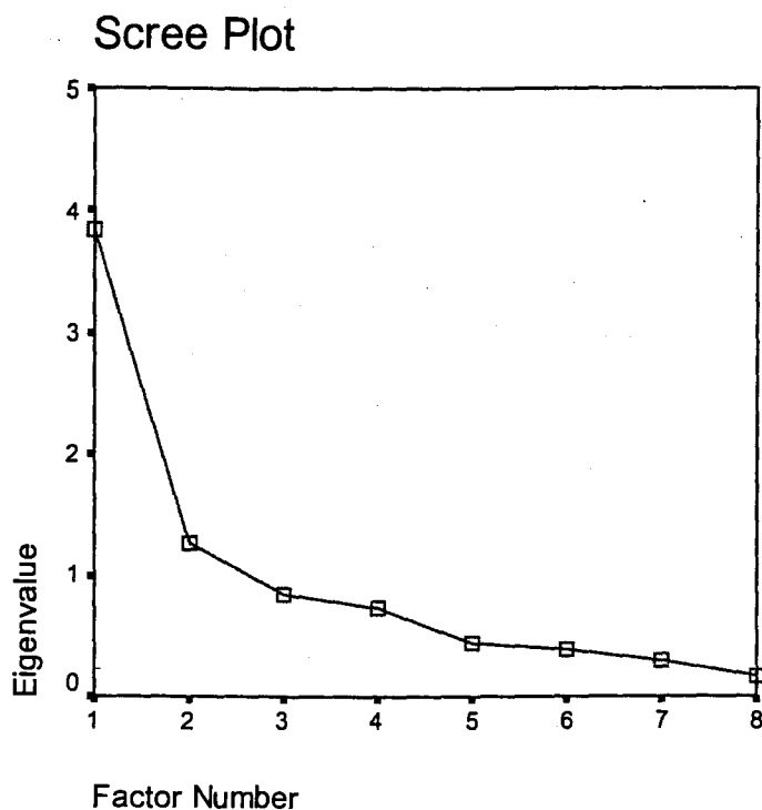
Figur 6.5 Scree plot Helse-, miljø- og sikkerhetsregler
